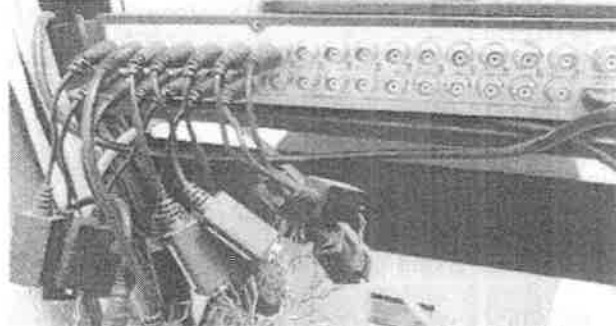
Imagen 2. Panel trasero que muestra la conexión de las 16 cámaras al DVR
